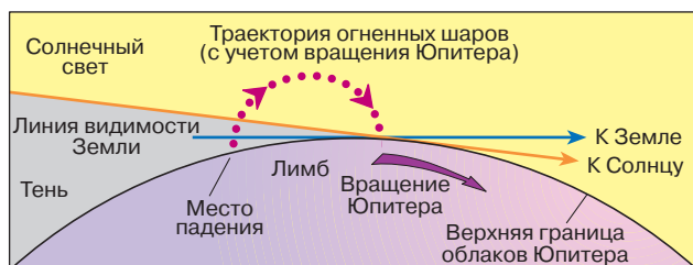
Рис. 2. Геометрия падения, вид сбоку. Падение происходило на теневой относительно Земли стороне Юпитера. Баллистические огненные шары-осколки вспыхивали за счет взрывной силы высвобождения кинетической энергии падения некоторых наиболее крупных фрагментов, которые сначала пересекали линию видимости Земли и затем вышли на солнечный свет. Через 10–30 мин осколки падали обратно в стратосферу на большой площади, производя сильное инфракрасное излучение, рассеяние осколков было видно многим наблюдателям
